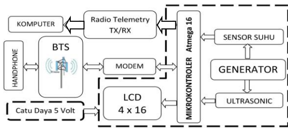
Gambar 9 Diagram blok sistem monitoring penggunaan (BBM) dan temperatur pada genarator
