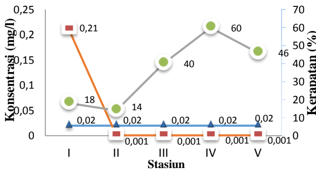
Gambar 3. Hubungan fosfat, nitrat dan kerapatan makrofita akuatik (Ket: ■ fosfat (mg/l); ▲ nitrat (mg/l); dan ● kerapatan (%)).
