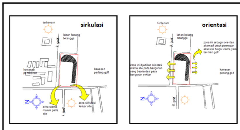
Gambar 5: Konsep Sirkulasi dan Konsep Orientasi club house alam khatulistiwa golf di Kota Pontianak
