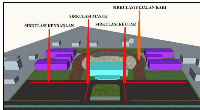
Gambar 7: Analisis dan Konsep Sirkulasi Rumah Edukasi Anak di Kota Pontianak
