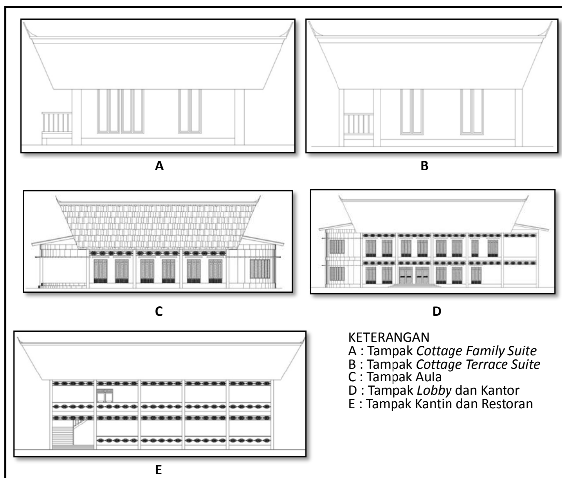
Gambar 12: Hasil Gubahan Bentuk Bangunan Perancangan Resort di Kecamatan Sungai Kakap Kabupaten Kubu Raya
