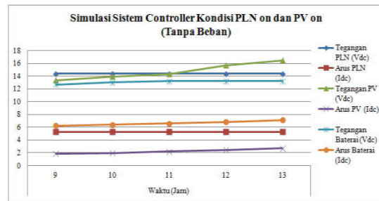
Gambar 10. Grafik Sistem Kendali Kondisi PLN on dan PV on (Tanpa Beban)
