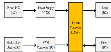
Gambar 3. Diagram Block Rancangan Simulasi Prototipe Pengendali PLN dan PV-system
