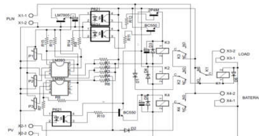
Gambar 4. Skematik Rancangan Simulasi Prototipe Pengendali PLN dan PV-system
