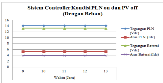
Gambar 6. Grafik Sistem Kendali Kondisi PLN on dan PV off (Dengan Beban)
