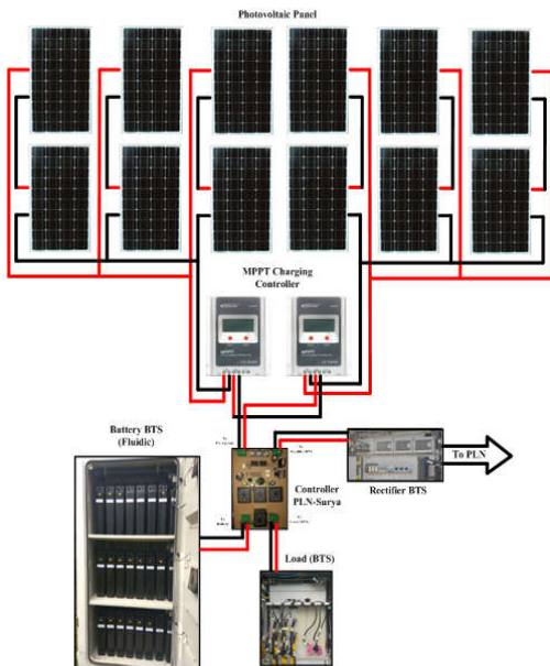
Gambar 13. Rancangan Wairing diagram Sistem Kombinasi Sumber Listrik PLN dan Energi Surya
