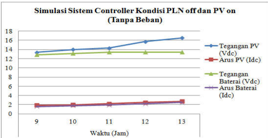
Gambar 7. Grafik Sistem Kendali Kondisi PLN off dan PV on (Tanpa Beban)
