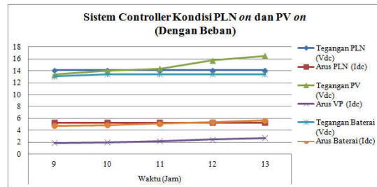
Gambar 11. Grafik Sistem Kendali Kondisi PLN on dan PV on (Dengan Beban)
