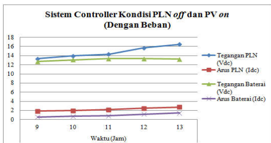
Gambar 8. Grafik Sistem Kendali Kondisi PLN off dan PV on (Dengan Beban)
