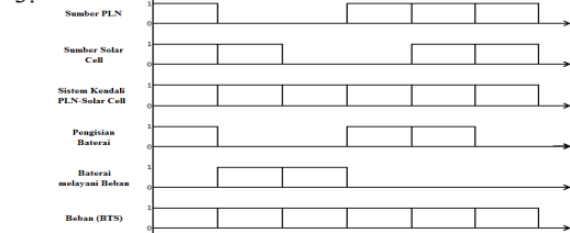
Gambar 2. Diagram State Rancangan Simulasi Prototipe Pengendali PLN dan PV-system
