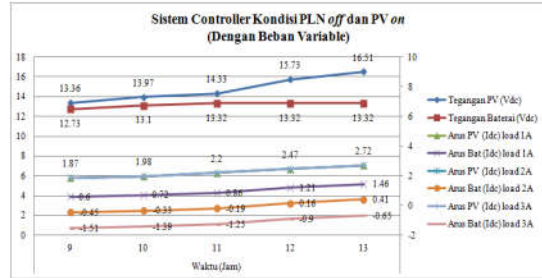
Gambar 9. Grafik Sistem Kendali Kondisi PLN off dan PV on (Dengan Beban Lampu 12V dan 1A ; 2A ; 3A)
