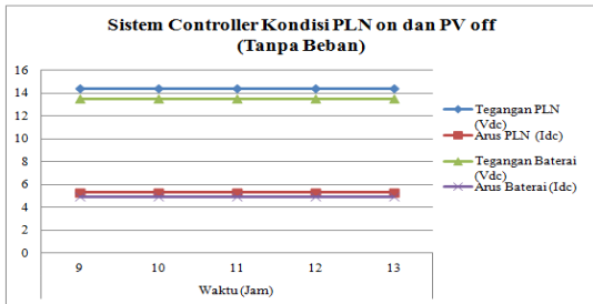
Gambar 5. Grafik Sistem Kendali Kondisi PLN on dan PV off (Tanpa Beban)
